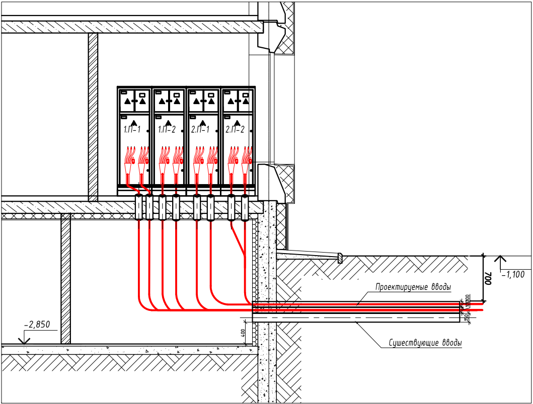
Разрез 1-1
